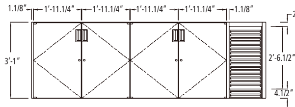
DOOR
